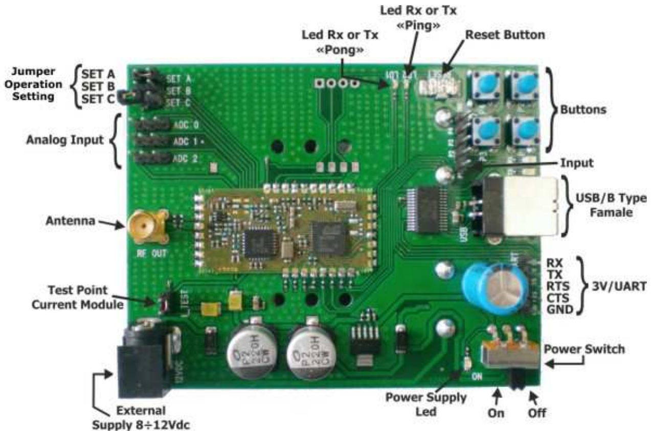
Figura 3: Descrizione lato top della demo XTR-8LR100/XTR-8LR10
