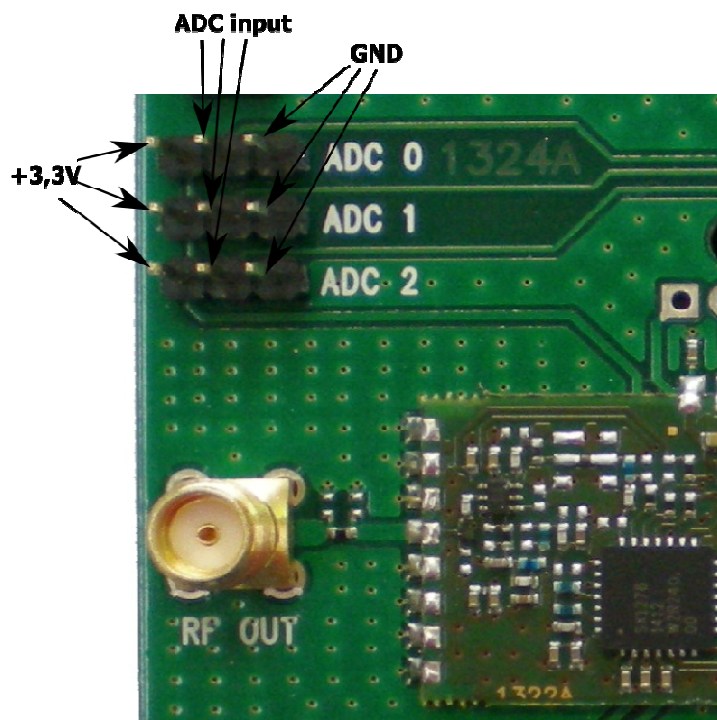
Input ADC disponibili su DEMO XTR-8LR100
